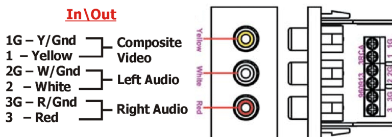
Цоколевка
