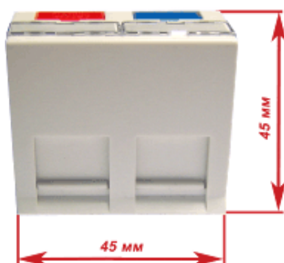
Insert Dimensions
